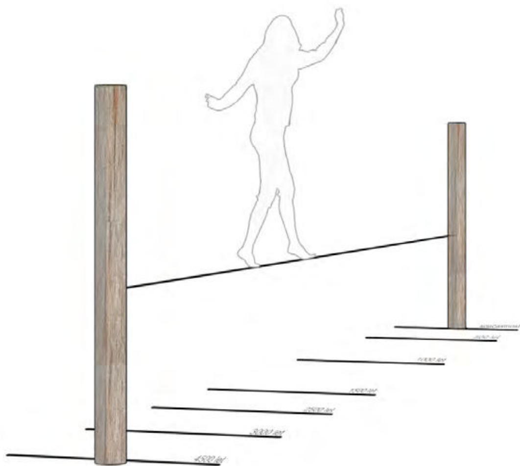
Slackline po geologických epochách
