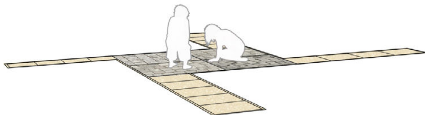
Křížovka z hornin
